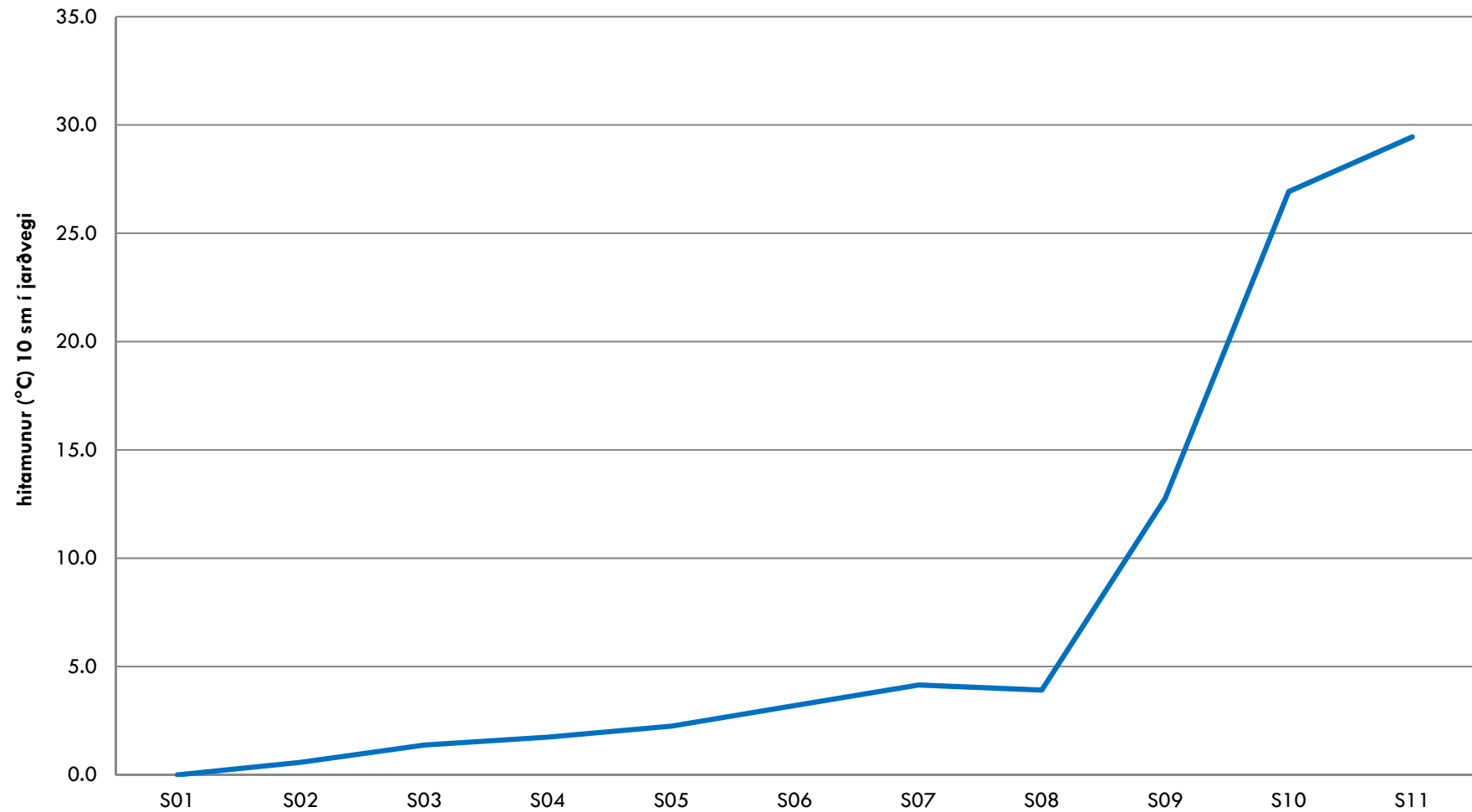
Meðal jarðvegshiti í skóglendi
