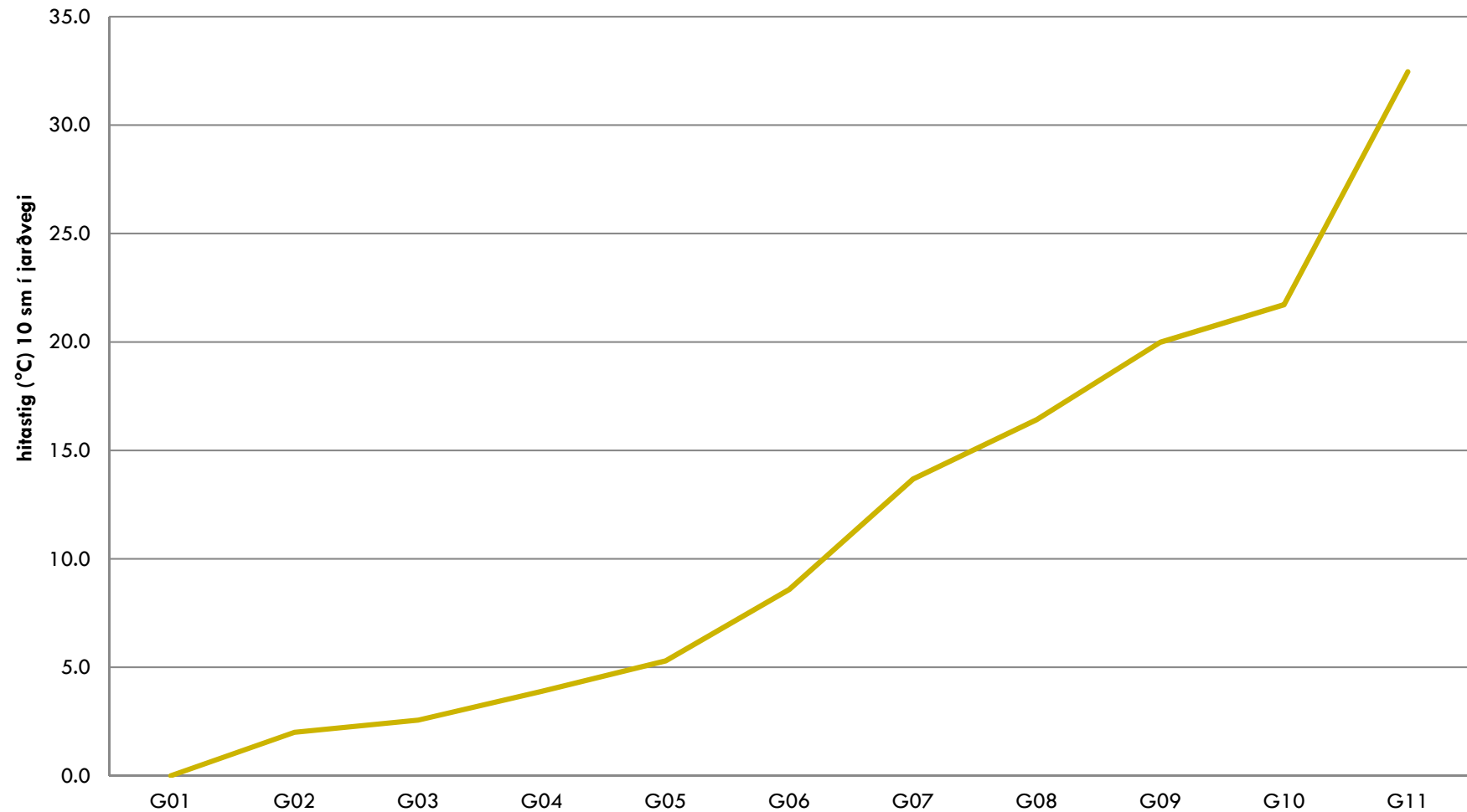
Meðal jarðvegshiti í graslandi
